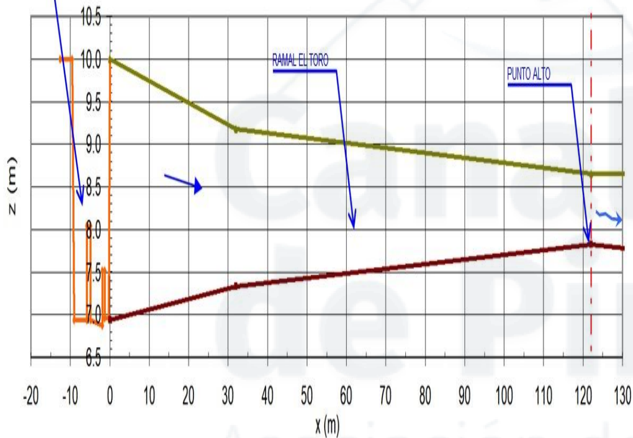
PERFIL CANAL LA SIRENA Y TOMA EL TORO
