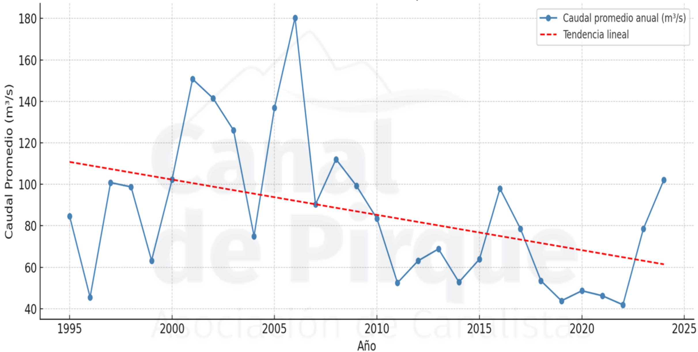
Tendencia del Caudal Anual del Río Maipo-La Obra (1995-2024)
